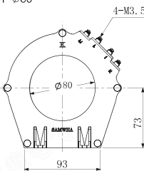
ZCT-Ø80
