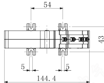
安装孔尺寸
