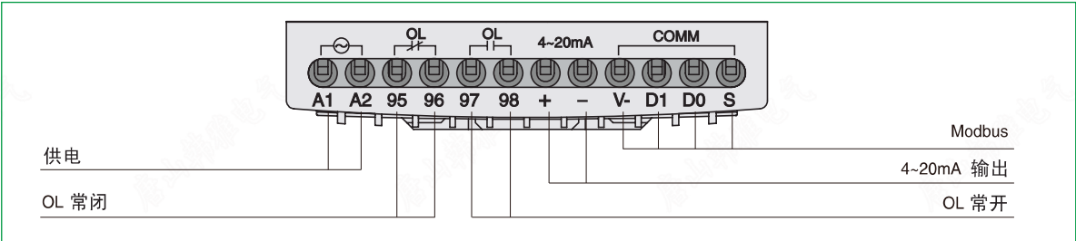
端子图
