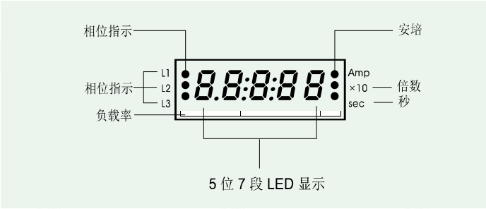
3相电流值2秒间隔循环显示
